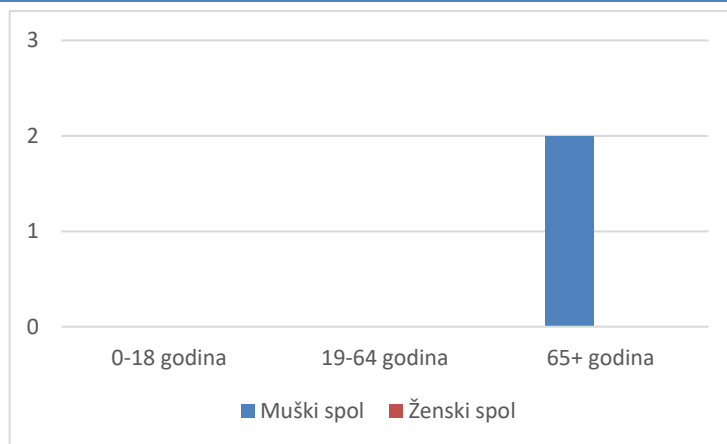
Grafikon 2. Spolna i dobna struktura preminulih u protekla 24 sata Prosječna dob smrtnih ishoda je iznosila 80,5 \pm 8,5
